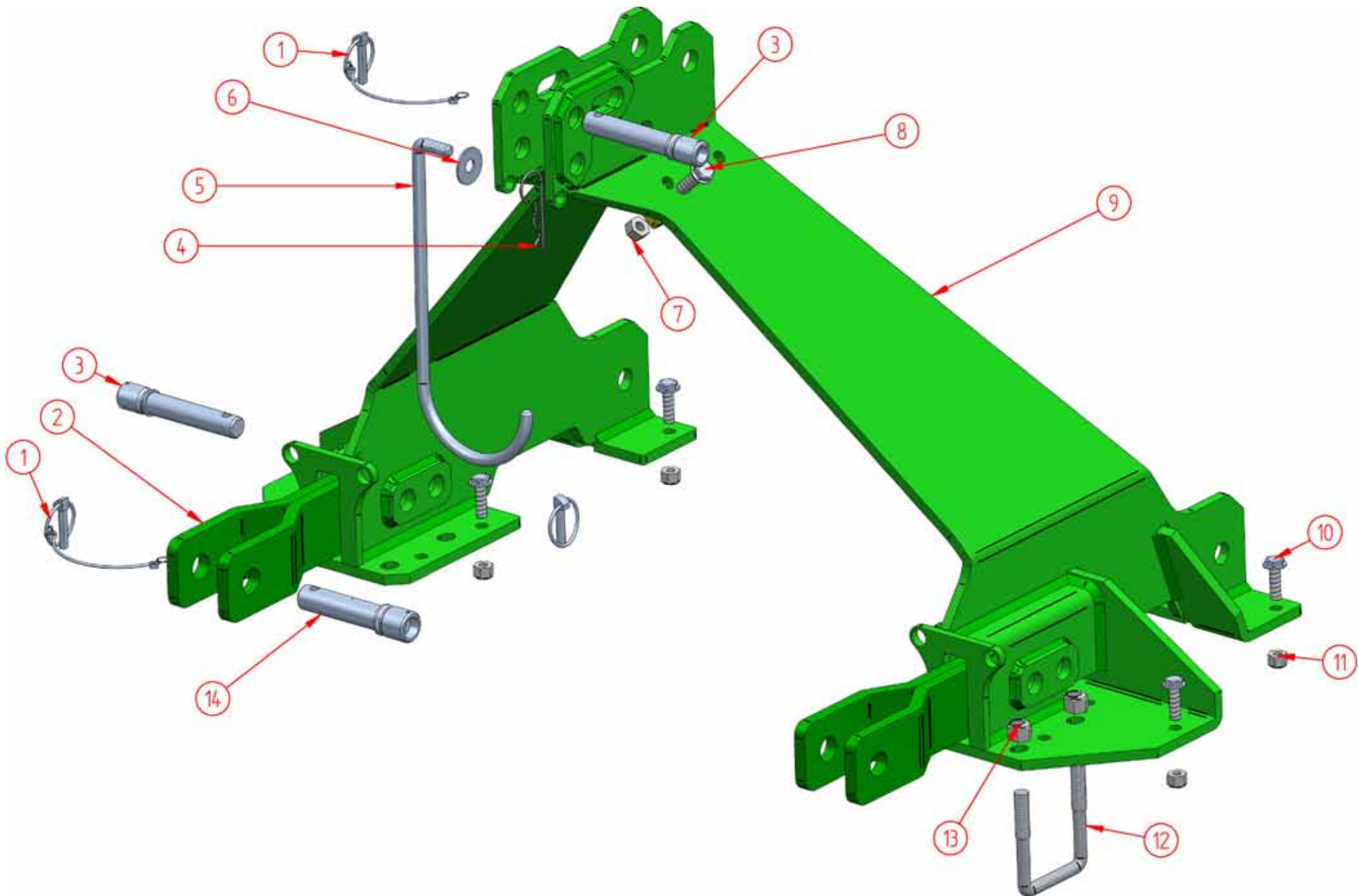
SERIE M.A. - KRONOS THIRD POINT LINKAGE
