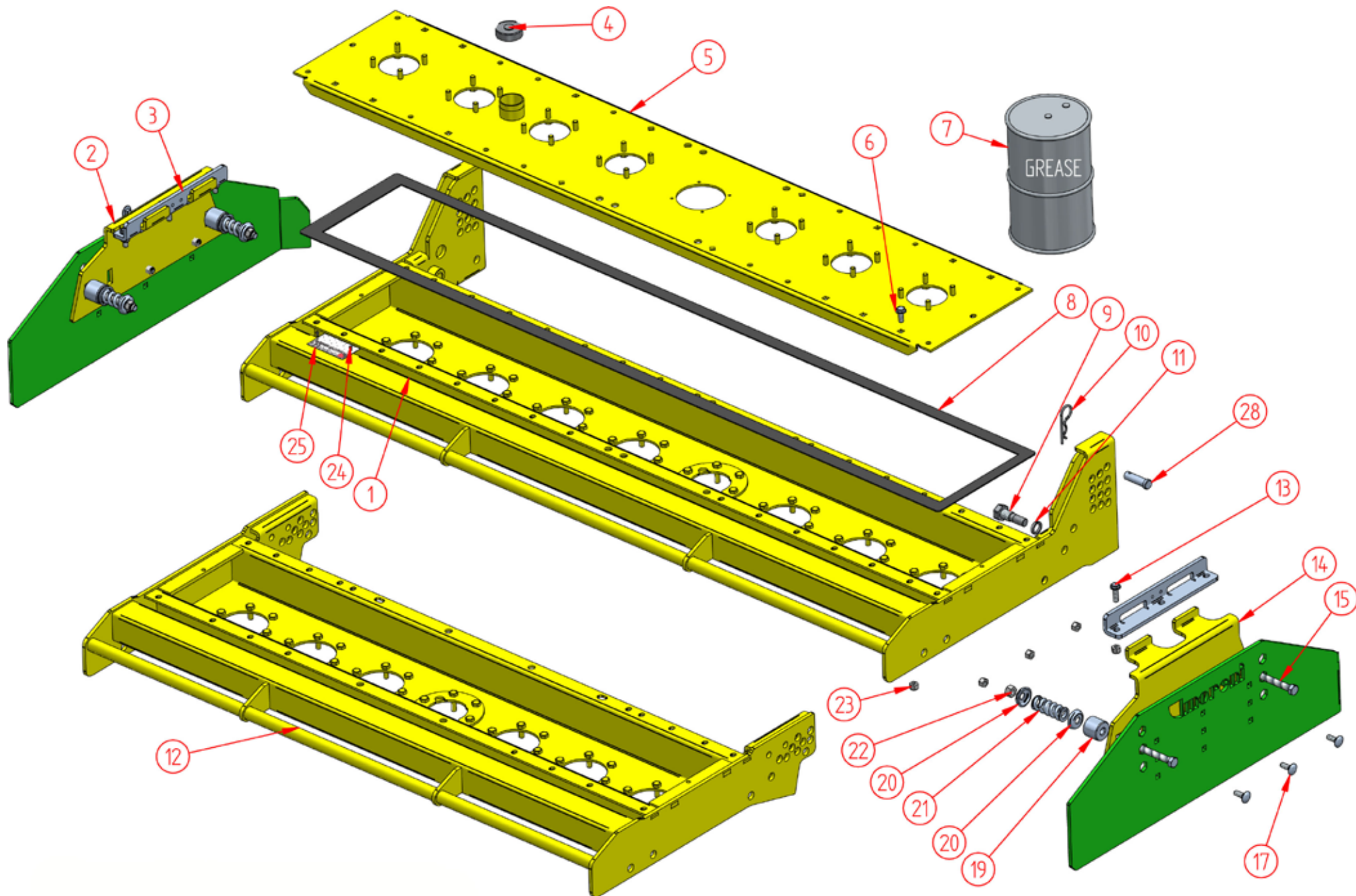
CASSAFORMA ERPICI FISSI - POWER HARROWS CASE
